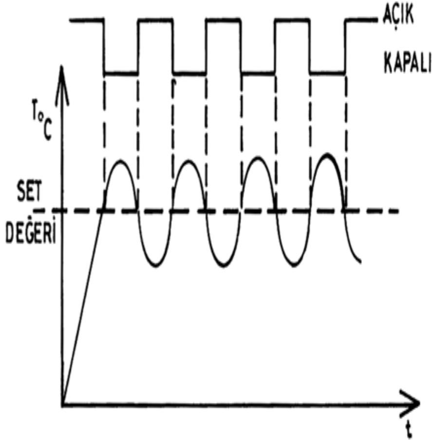
Açık-kapalı kontrol (ideal)
