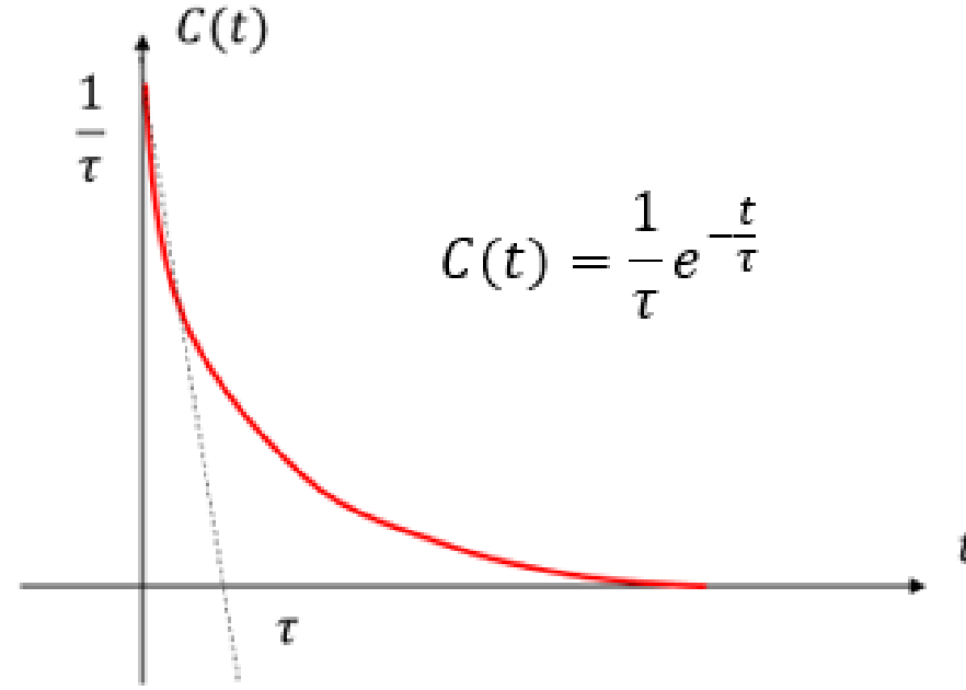
Şekil 6.6 Birim impuls yanıtı
