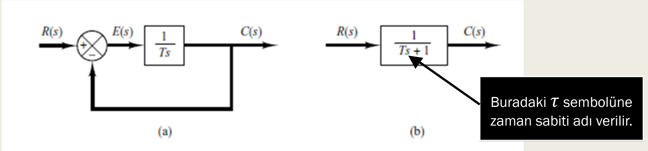
Şekil 1 (a) Birinci dereceden bir sistemin blok diagramı (b) Basitleştirilmiş blok diyagram
